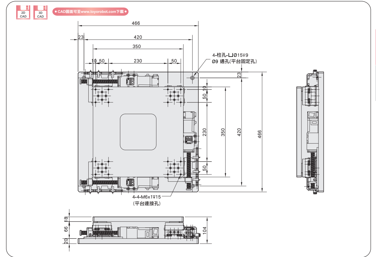
EXYY-035-035-M10 尺寸圖 Size
