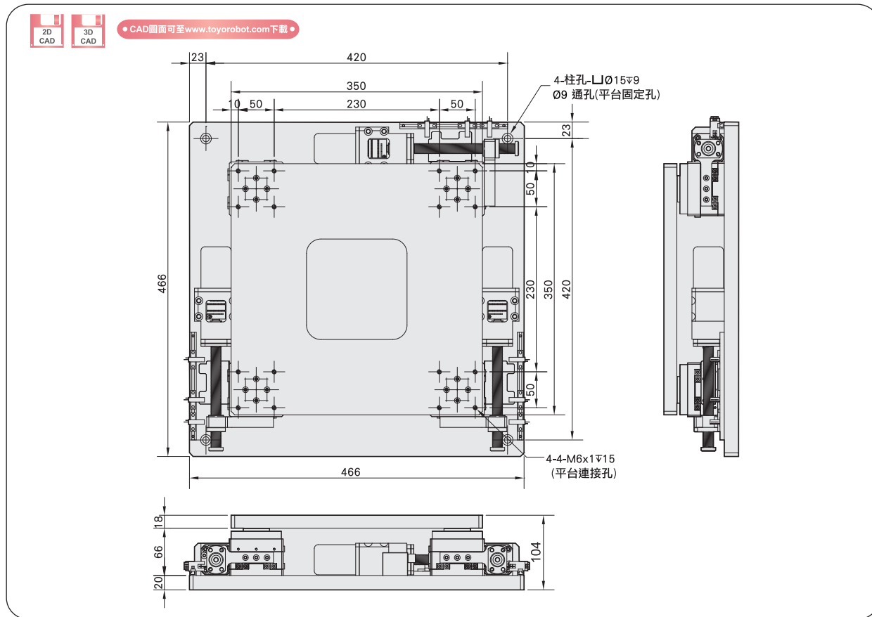
EXYY-035-035-42M 尺寸圖 Size
